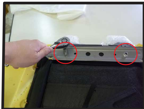
⑥背もたれを裏返し、アームレストを固定しているナットを、ラチェット等を使用し外します。
