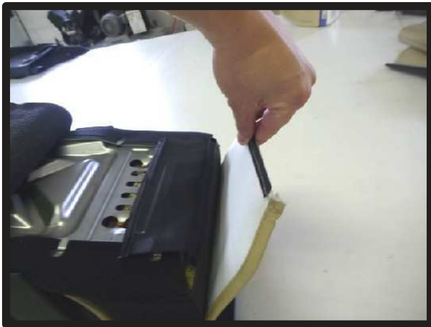
⑧アームレスト裏側へ生地を引き出します。
