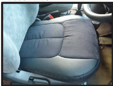
⑱カバーのラインを整えて運転席側座面の完成です。助手席側も同様に取り付けます。
