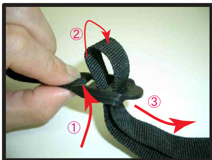
⑯ベルトは①→②→③の手順で、まずバックル中央を通し、折り返してバックルの端に通します。通したベルトを引くとカバーの前後を引き絞り固定されます。
