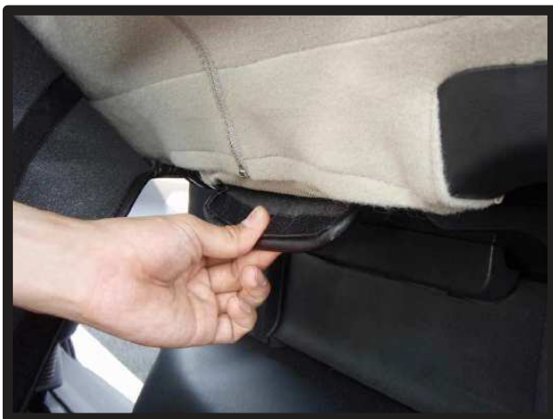
⑨座面を跳ね上げ、③で入れ込んだ生地を引き出します。
