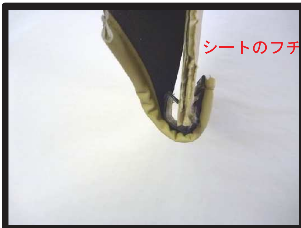
⑮折り返したフックを下から上へ引っ掛けるようにして、シートのフチに固定します。
