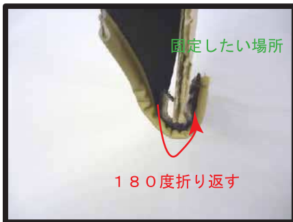
④プラフックは、生地と共に180度折り返し、固定したい場所に下から上へ引っ掛けるようにします。 ※図は、固定したい場所を仮に表しています。
