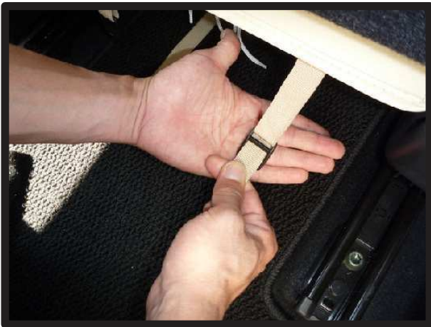
⑮引き出したベルトを1ページの④で引き出した生地についているバックルに通して固定します。
