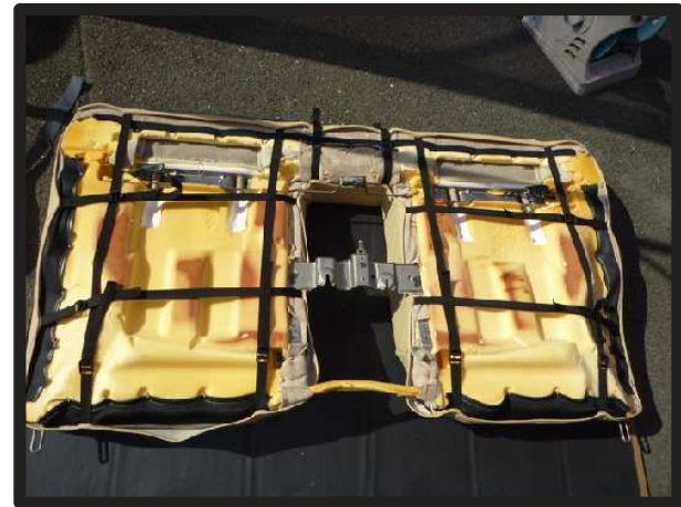
⑭背もたれを裏返して、カバーの上下左右に付いているベルトで固定します。
