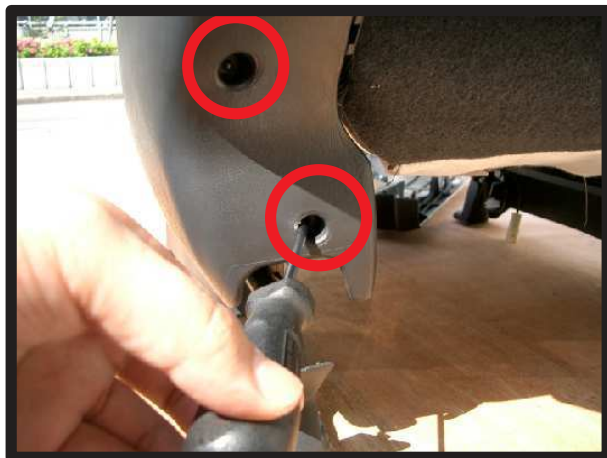
④カバー後ろについているネジもはずして下さい。
