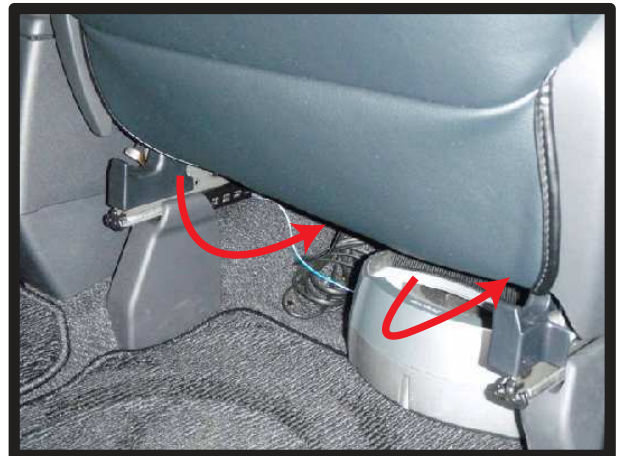
⑪ 背もたれから座面下を覆うカバーにゴムがありますので、S字フックを取り付け、座面下の適当な金属部分に引っ掛けます。
