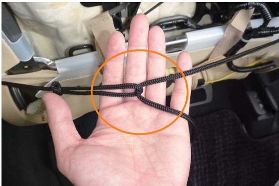
7 カバー両側面に付いているヒモの一方で輪を作り、もう一方を輪に通します。
