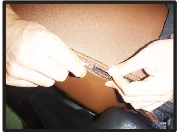
⑩背面のファスナーを生地を内に寄せながら閉じます。 ファスナーの先端はカバーの中へ入れ込みます。
