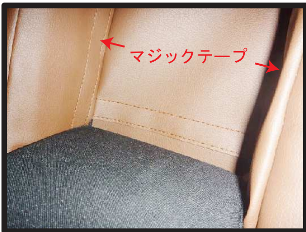
㉓ アームレスト収納部のマジックテープをシートに直接固定します。
